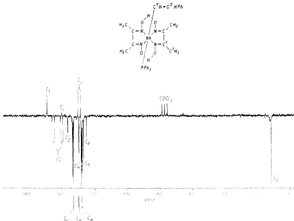
Fig. 1. APT- ^{13}\text{C}\{^1\text{H}\} -NMR-Spektrum von \text{Rh}(\text{PPh}_3)(\text{dmgH})_2(\text{CH}=\text{CHPh}) (IV) in \text{CDCl}_3 als Lösungsmittel (positiv: quaternäre C-Atome; negativ: sekundäre und tertiäre C-Atome).
